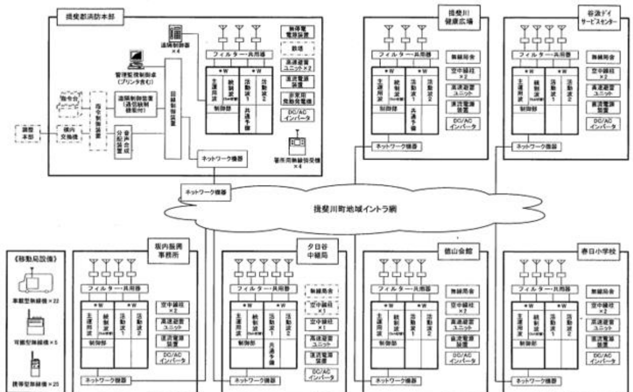
消防救急デジタル無線×システム系統図
